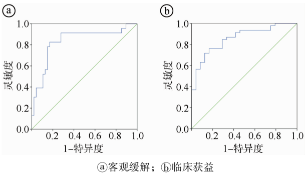
图 1 血清 TRAIL 水平预测 NSCLC 患者免疫治疗反应的 ROC 曲线图
