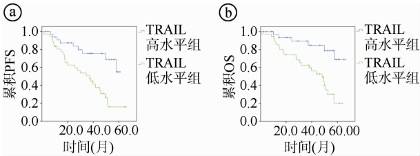
图 2 TRAIL 低水平组和 TRAIL 高水平组的 Kaplan-Meier 曲线比较
